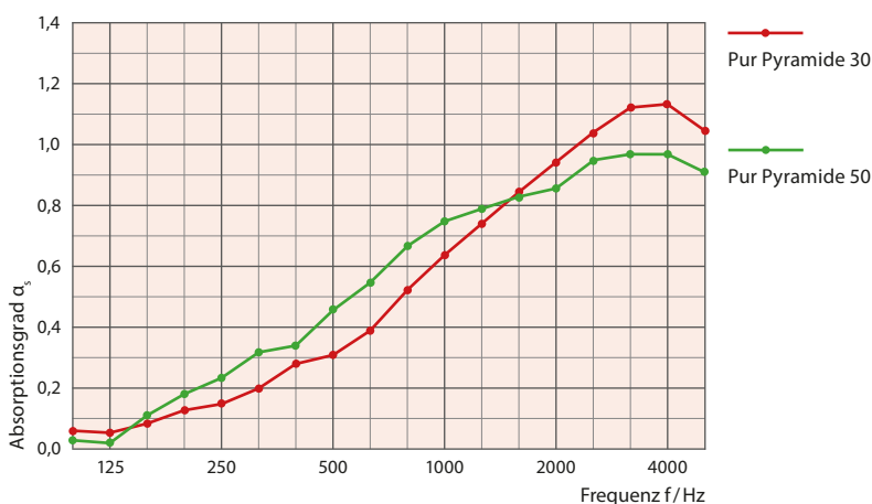
Labor-Messung in Anlehnung an ISO 354:
